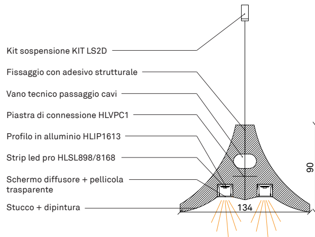
Piastra di connessione HLVPC1
